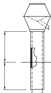
Tipo ARI per tetto piano
